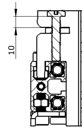
SECTION B-B SCALE 1 : 2
